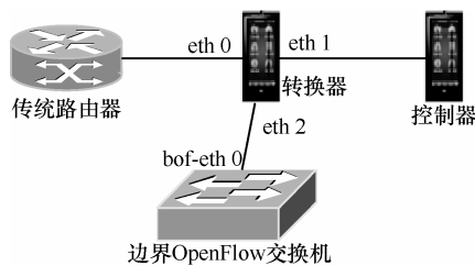
图 2 转换器连接
