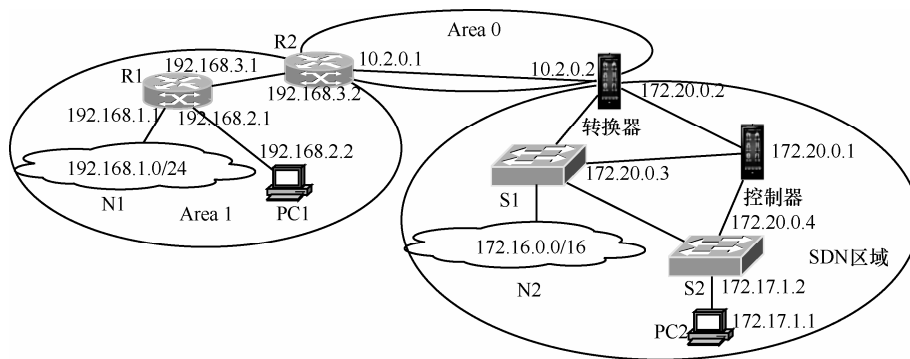
图 4 IMISA 架构部署网络拓扑
