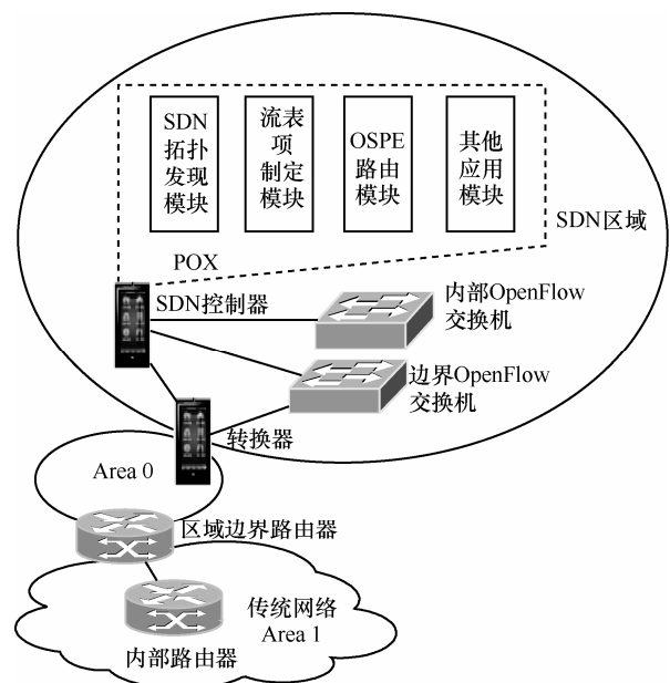
图 1 IMISA 总体架构
