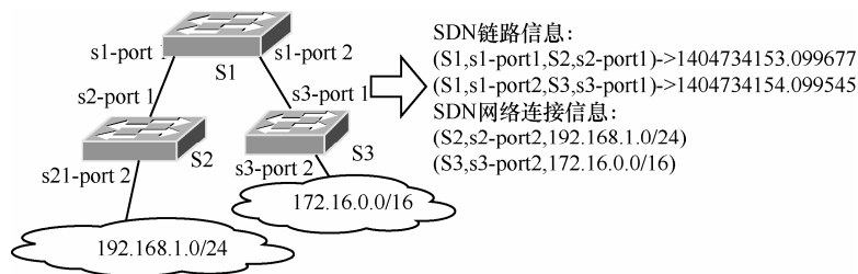
图 3 网络拓扑与存储信息映射
