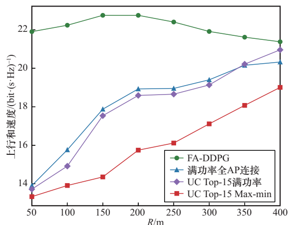
图6 不同方案下上行和速率随轨道半径的变化关系
