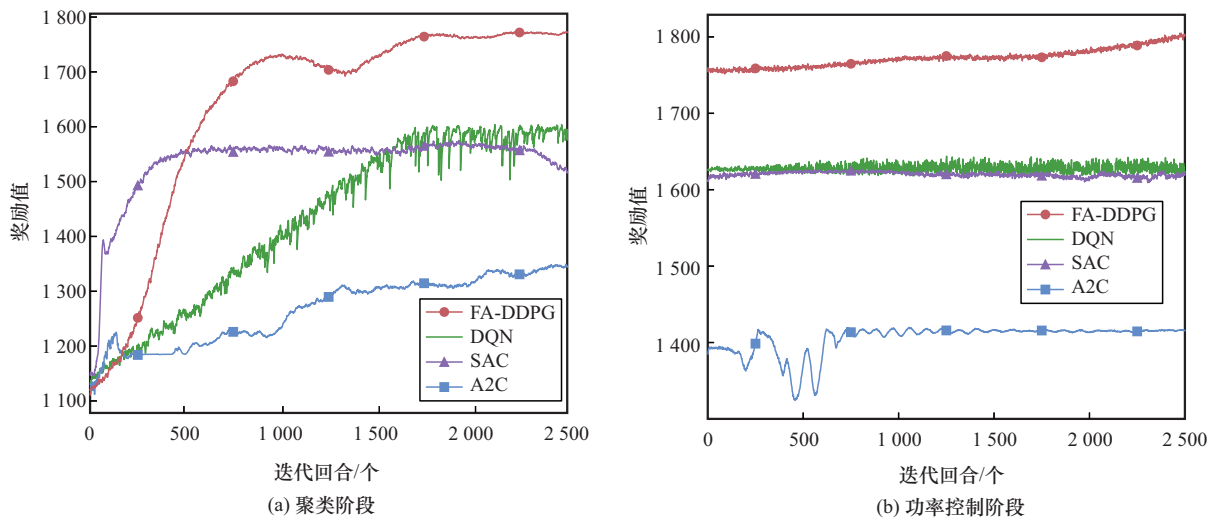
图3 不同RL算法的训练回报
