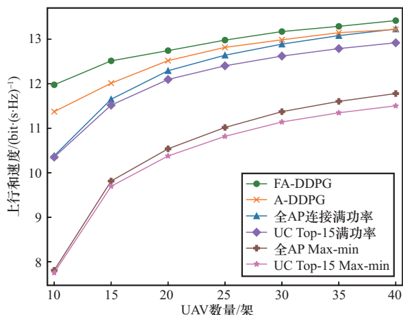
图4 不同算法的上行和速率与UAV数量的关系
