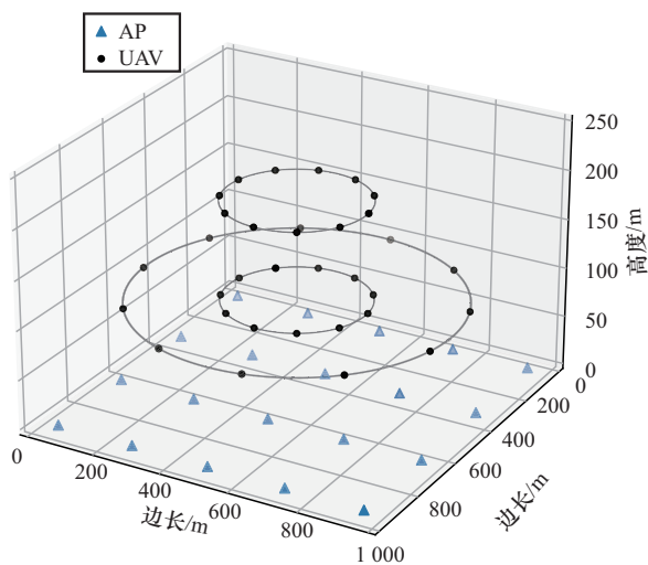
图5 UAV飞行轨迹
