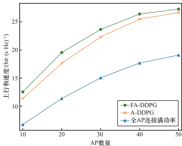
图7 不同方案下上行和速率随AP数量的关系
