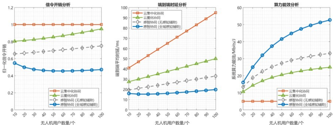
图4 不同协同方式通算融合网络性能分析
