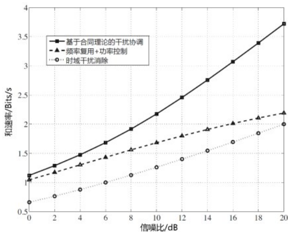
图7 通信计算融合无线网络干扰协调算法性能 转载自[36]图4.5
