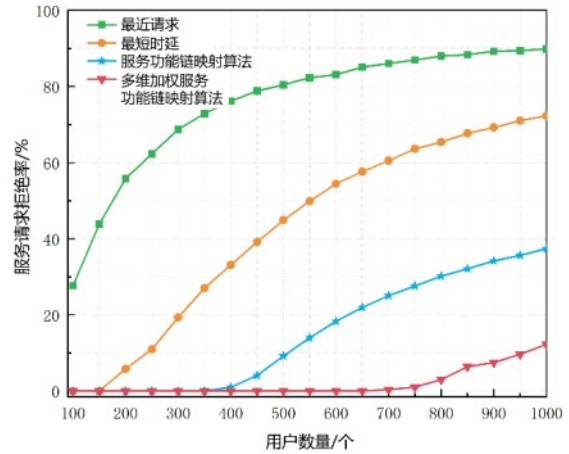
图9 基于切片的服务请求拒绝率 转载自[50]图3
