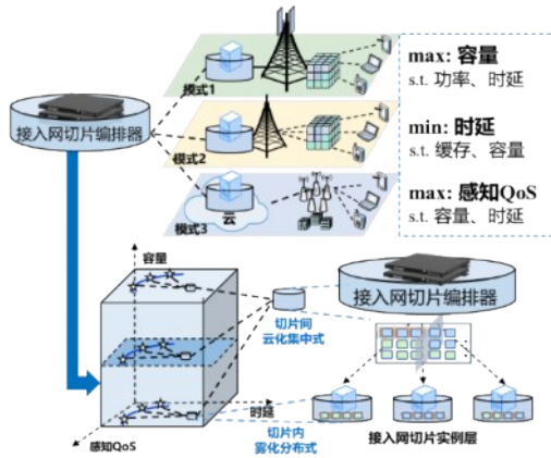
图8 通信计算融合无线网络云化协同通算资源调度
