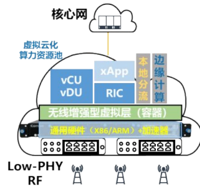
图6 云雾化协同网络架构
