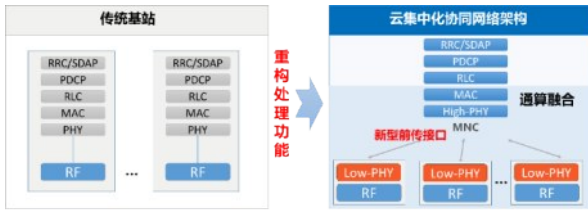
图5 云集中化协同网络架构
