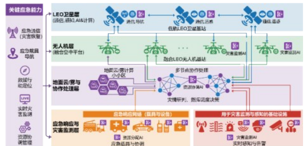
图 15 面向应急场景应用的感知协同组网
